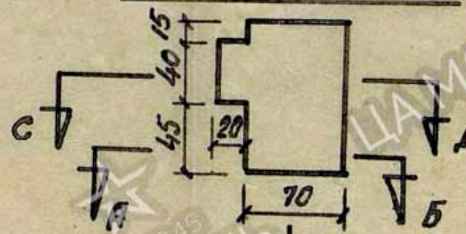
Вид амбразур
