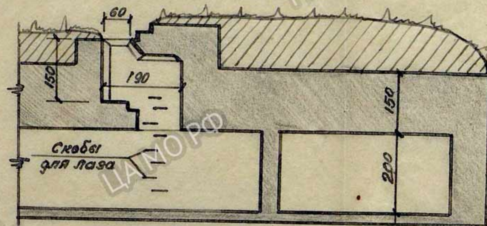
Разрез по С-Д
